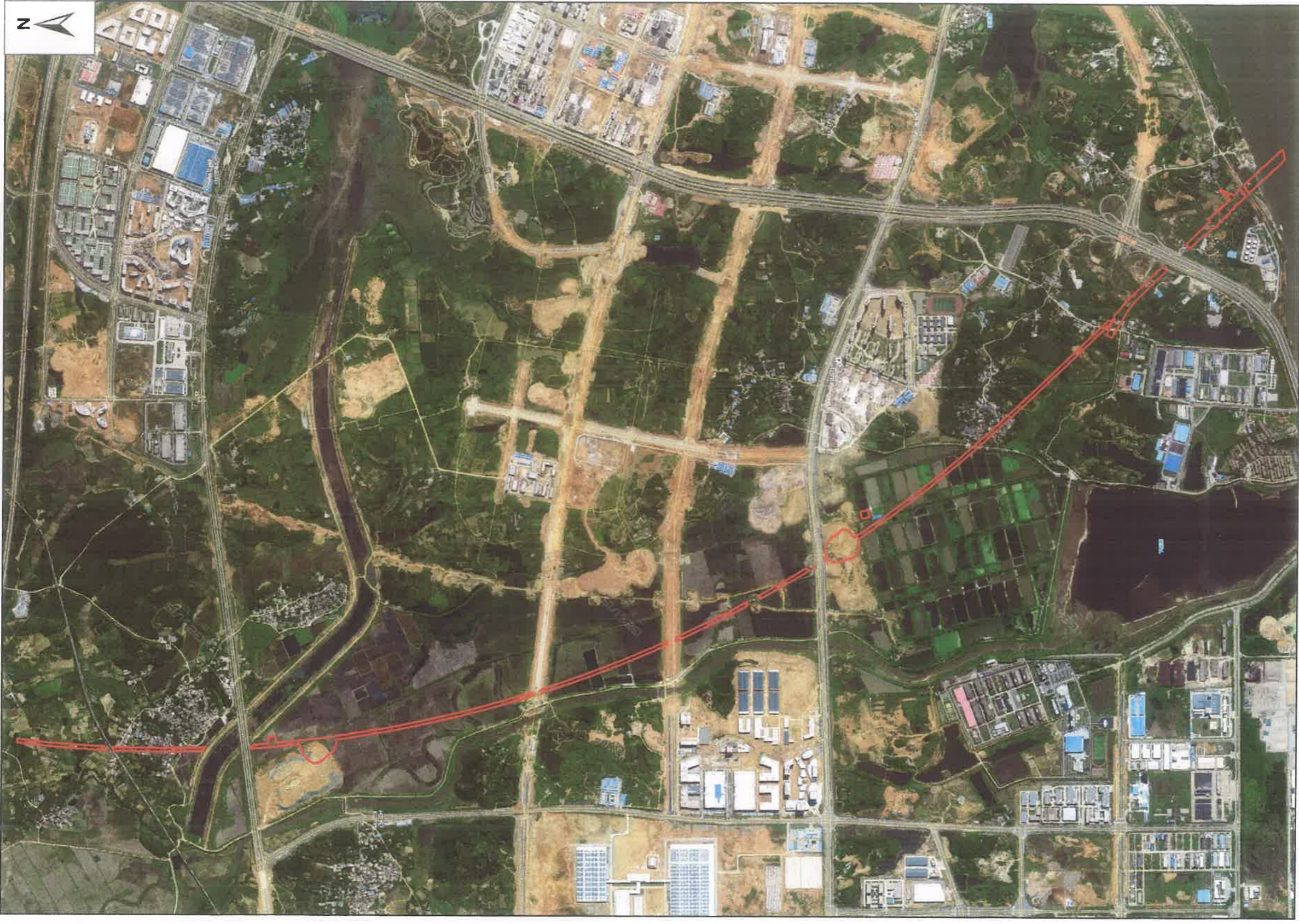
新建京港高速铁路九江至南昌段涉及南昌经济技术开发区征地区红线图
